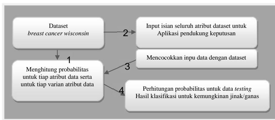
Gambar 4 Alur aplikasi
