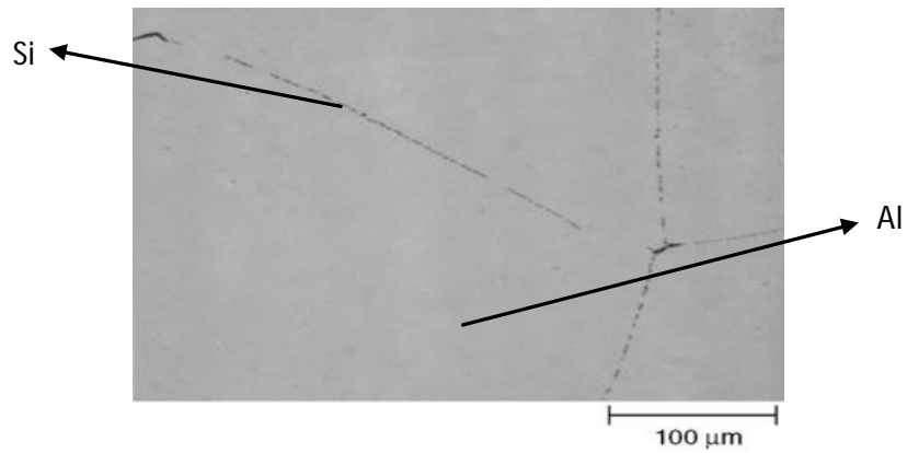
Gambar 4. Struktur mikro kawat aluminium (200x)
