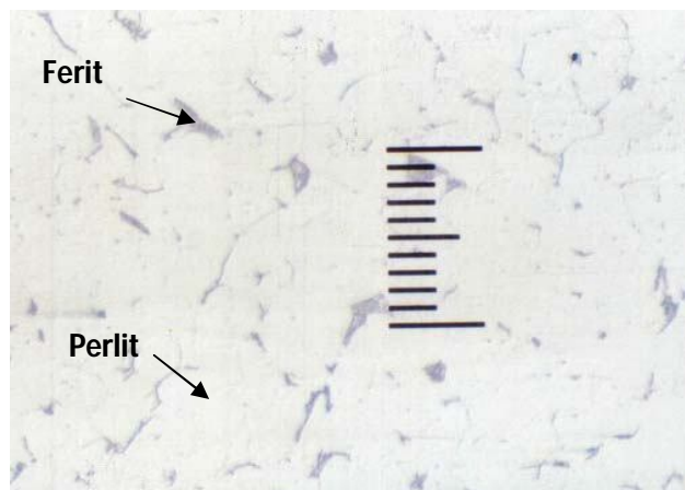
Gambar 5. Struktur mikro permukaan pipa baja galvanis
