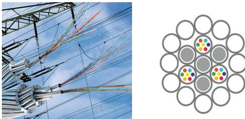
Gambar 3. Susunan kabel OPPC
