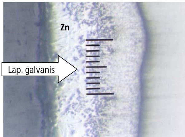
Gambar 6. Struktur mikro lapisan galvanis bagian dalam Pipa
