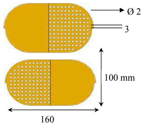
Gambar 1. Dimensi Katalis
