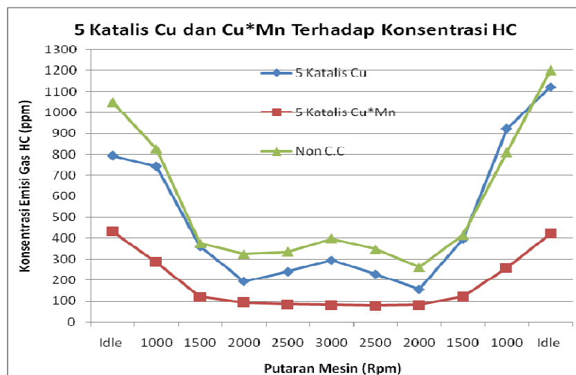
Gambar 8. Grafik Penurunan Emisi HC dengan 5 Sel Katalis
