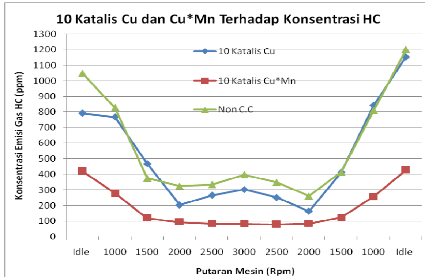
Gambar 9. Grafik Penurunan Emisi HC Dengan 10 Sel Katalis
