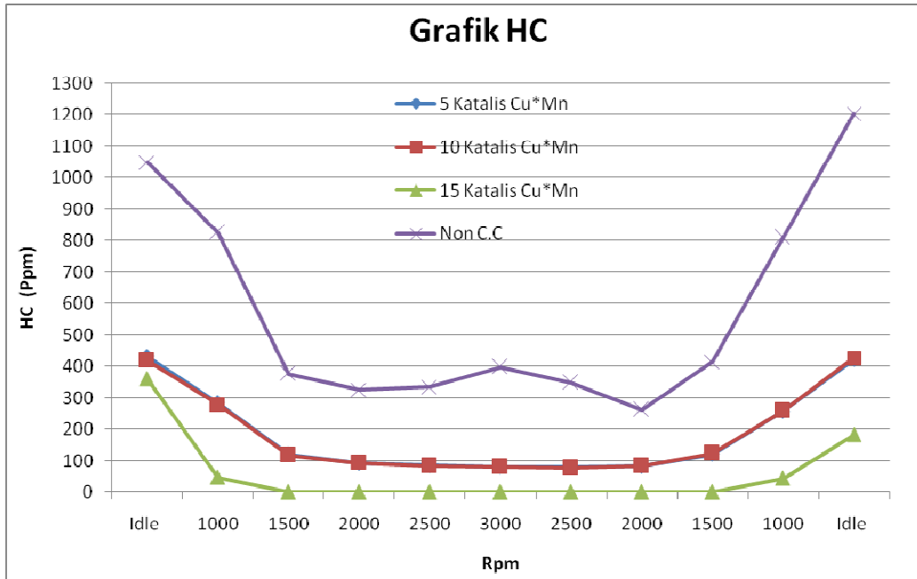
Gambar 11. Grafik Penurunan Emisi HC Dengan Tembaga Berlapis Mangan
