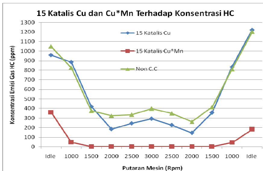
Gambar 10. Grafik Penurunan Emisi HC Dengan 15 Sel Katalis
