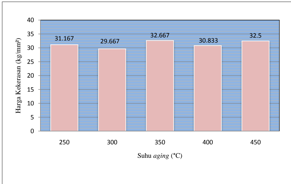
Gambar 1. Grafik hubungan antara suhu aging dan kekerasan. (kekerasan raw material = 35,5 kg/mm 2 )
