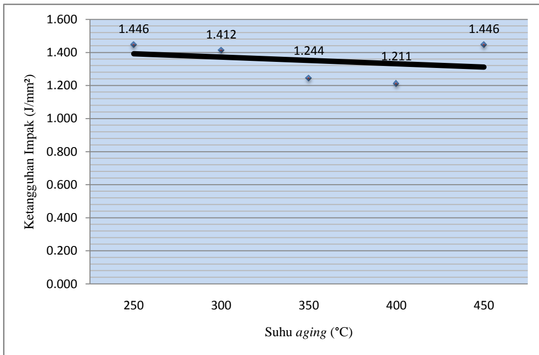
Gambar 4. Grafik trendline hubungan antara suhu aging dan ketangguhan impak
