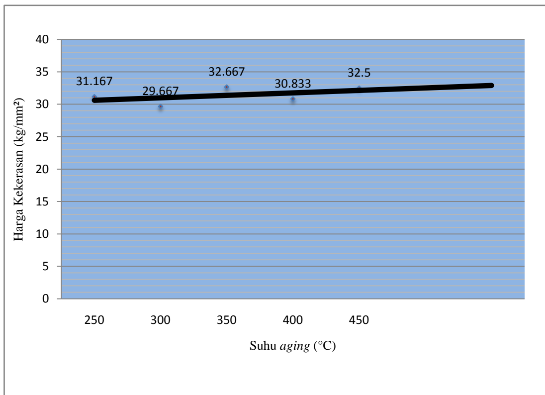
Gambar 1. Grafik hubungan antara suhu aging dan kekerasan. (kekerasan raw material = 35,5 kg/mm 2 )
