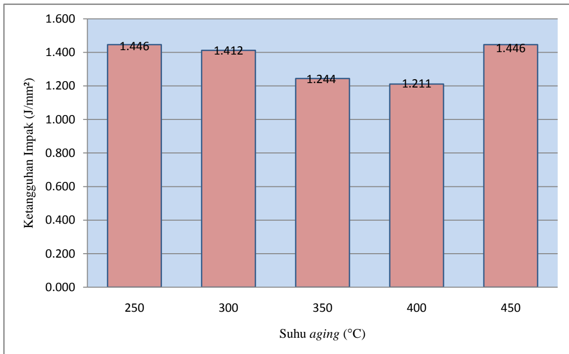
Gambar 3. Grafik hubungan antara suhu aging dan ketangguhan impak (ketangguhan impak raw material = 1,278 joule/mm 2 )
