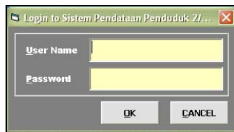
Gambar 20 : Form Login
