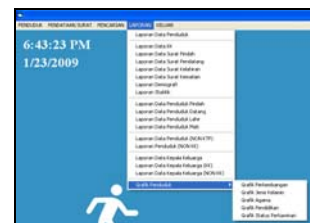
Gambar 26 : Menu Laporan
