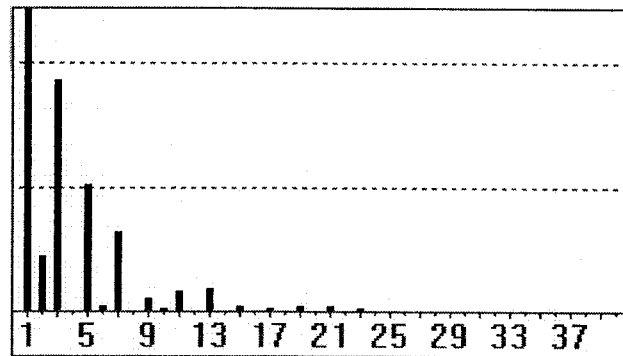
Gambar 2. Spektrum harmonisa
