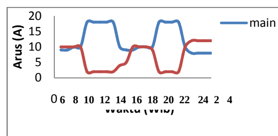
Gambar 9. Grafik Beban Nyata Terhadap Ballast Load hari Minggu.
