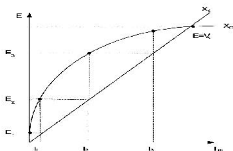
Gambar 1. Proses pembangkitan Tegangan
