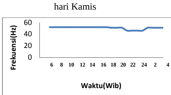
Gambar 11. Grafik perubahan frekuensi
