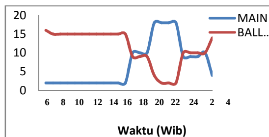
Gambar 8. Grafik Beban Nyata Terhadap Ballast Load hari Kamis.
