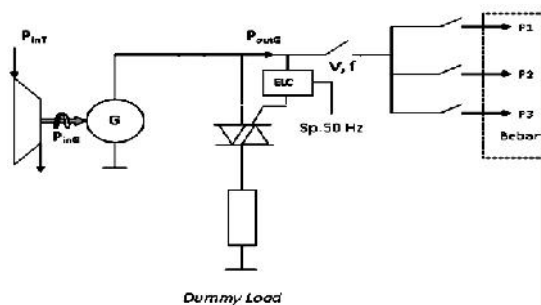
Gambar 6. Model kontrol beban pada PLTMh.
