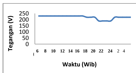
Gambar 10. Grafik Output Tegangan pada
