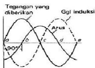
Gambar 4. Arus, tegangan dan GGL induksi-diri pada beban induktif
