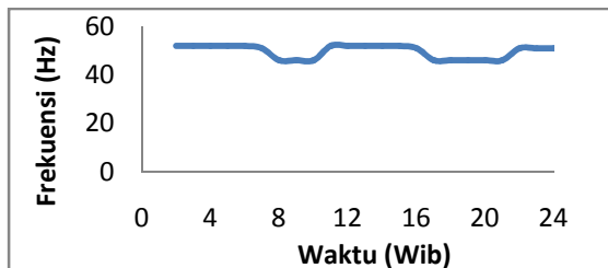
Gambar 13. Grafik Stabilitas Frekuensi Generator hari Minggu
