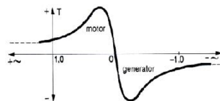
Gambar 2. Kurva karakteristik mesin induksi.
