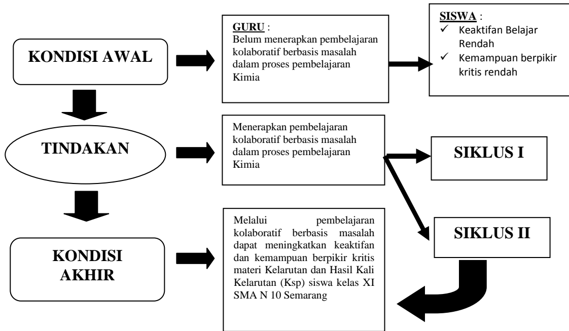
Gambar 1. Kerangka Berfikir
